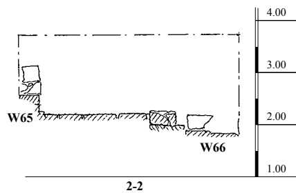
תכנית 1. שטח A, תכנית והתכים.
